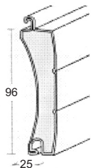
Alu lamela PA 96 (valjana alu pločevina)
